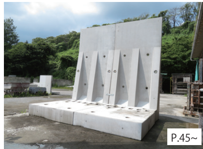
N-SKH 大型L型擁壁(オールプレキャストタイプ)
