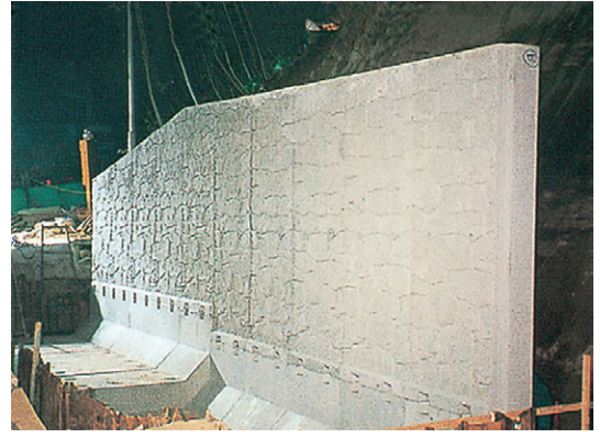
組立式逆L型擁壁 (H=6,200mm)
